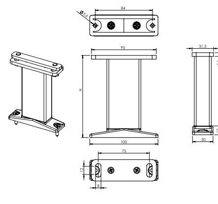
Držák VL Cv (2-01412-PU11X)
